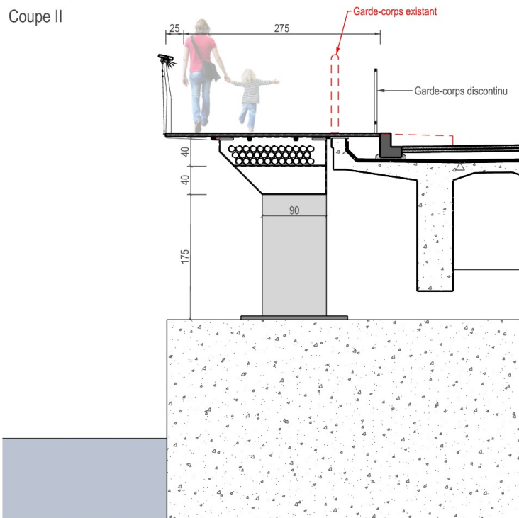
Coupe II
