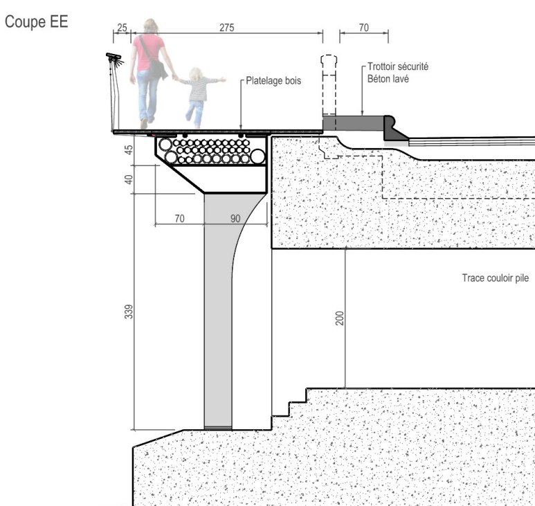
Coupe EE
