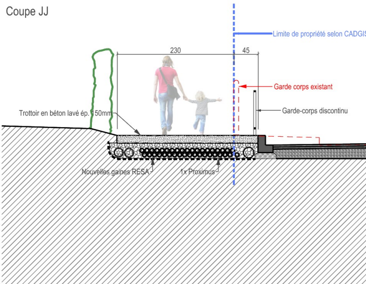
Coupe JJ
