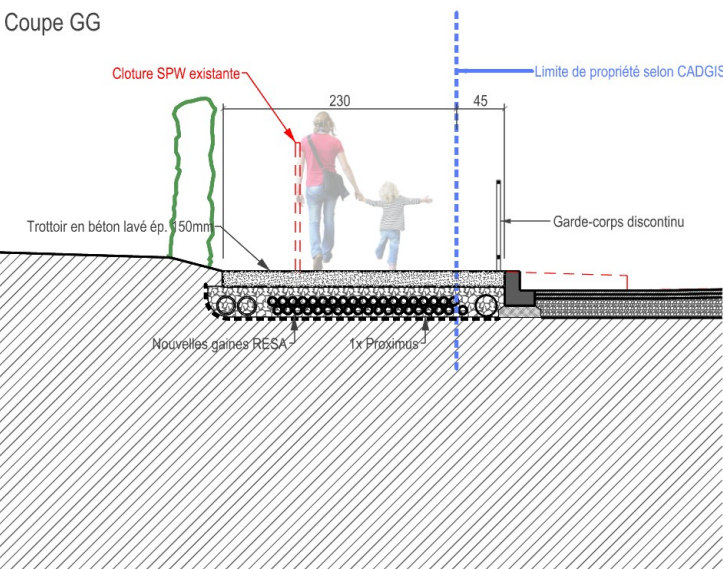
Coupe GG
