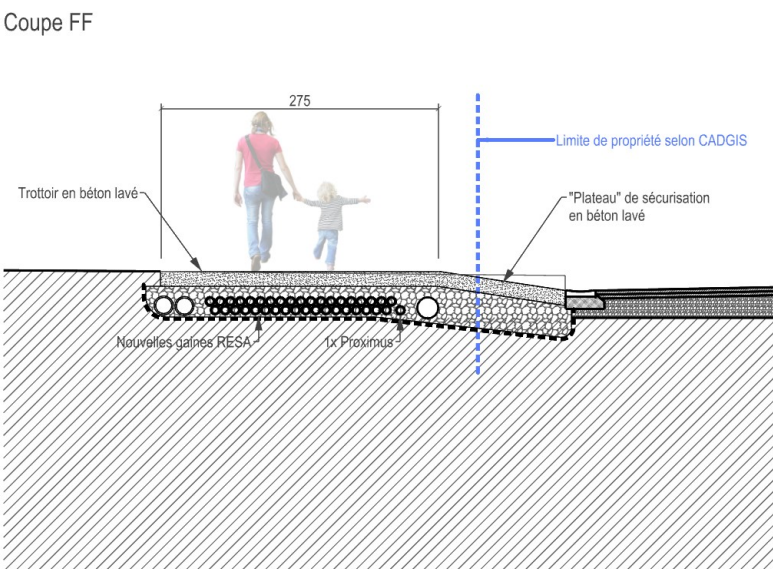
Coupe FF
