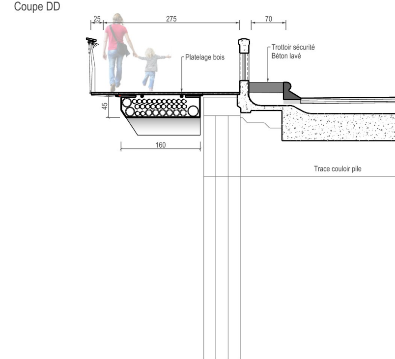
Coupe DD
