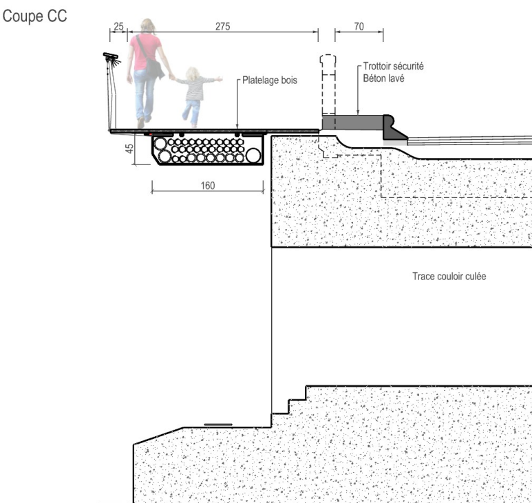
Coupe CC
