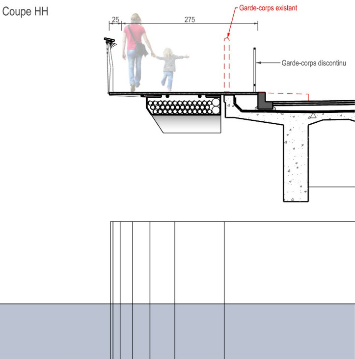
Coupe HH
