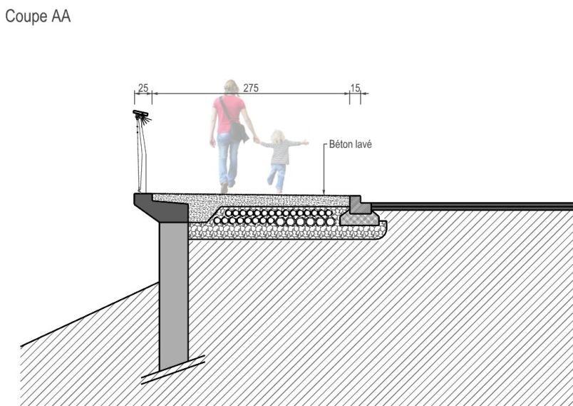
Coupe AA
