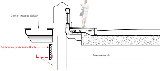
3- Tirage impétrants + suppression ancien chemin de cable
