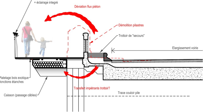
5- Pose trottoir en encorbellement + élargissement voirie
