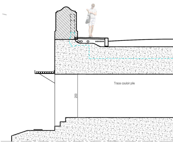
Coupe EE - Phasage de démolition
