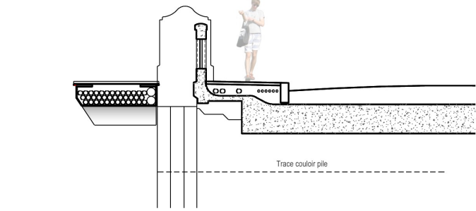
5- Pose trottoir en encorbellement + élargissement voirie
