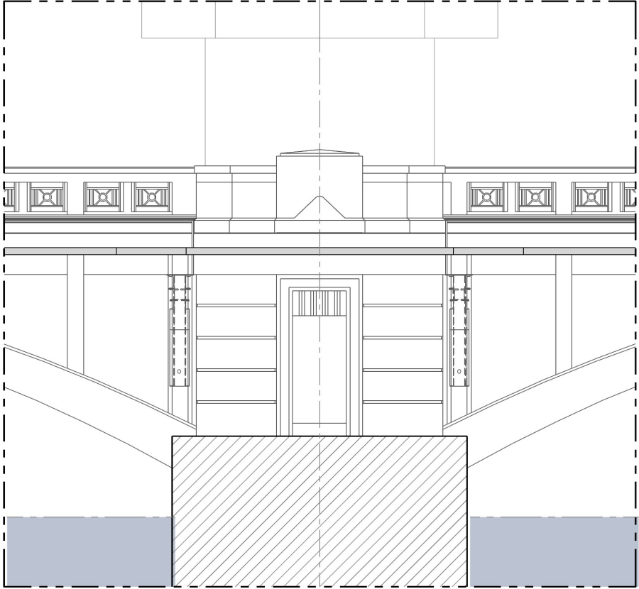
Elévation - Phasage de démolition
