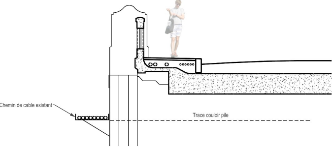
2- Pose nouveau chemin + déplacement provisoire existant
