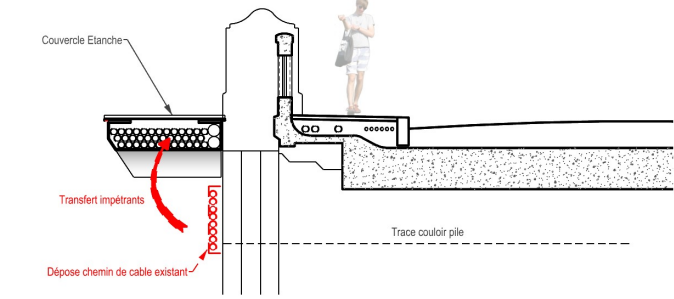
4- Situation définitive intermédiaire (couverture)
