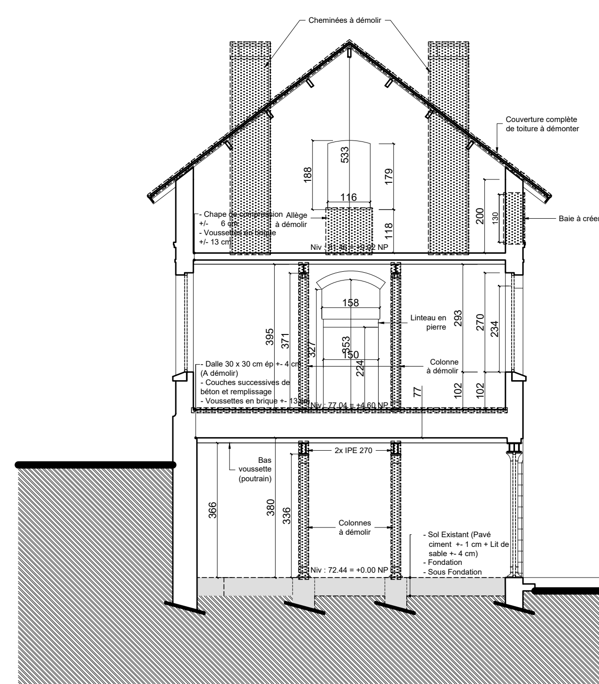
Coupe AA
