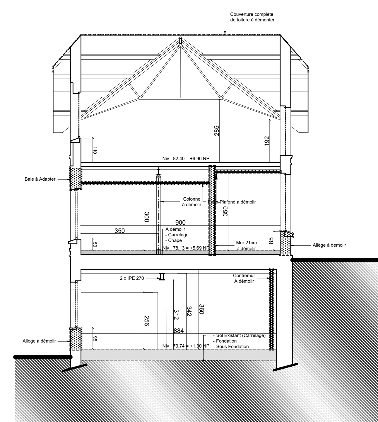
Coupe BB
