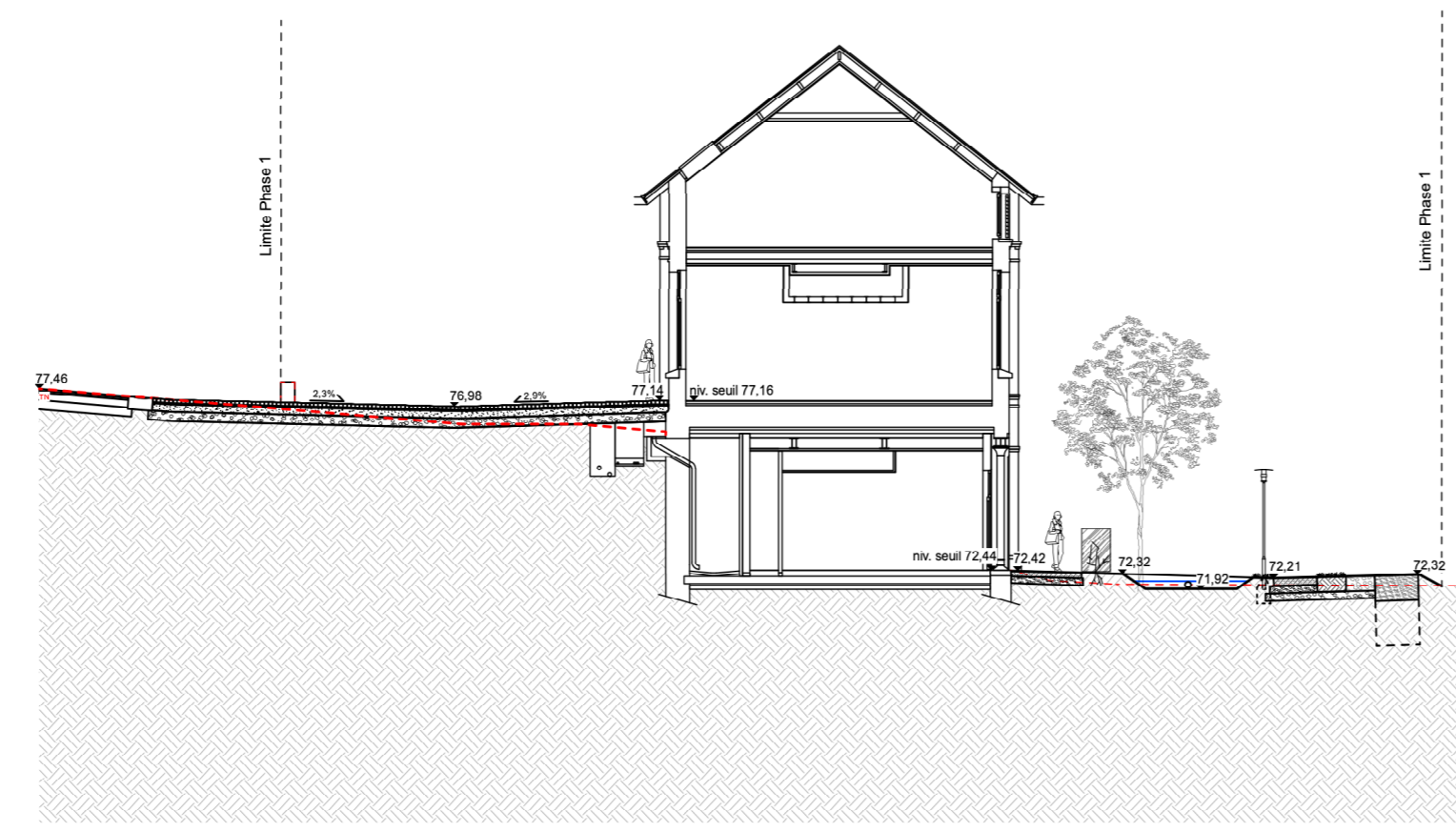
COUPE 2-2' échelle 1:200
