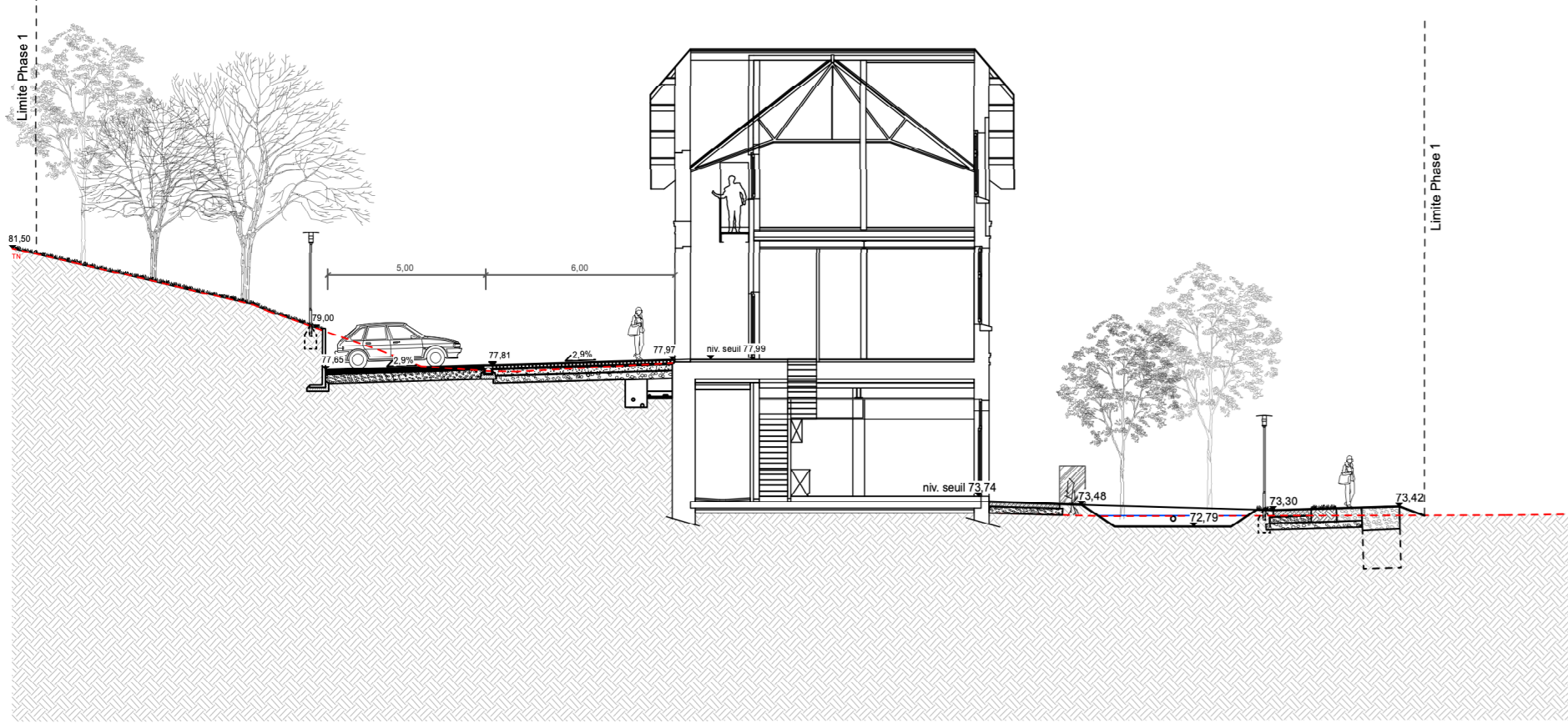
COUPE 1-1' échelle 1:200
